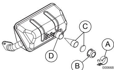
Figure 4-6. Écran pare-étincelles
