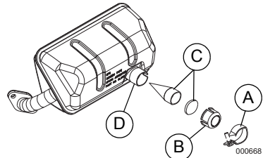
Figura 4-6. Tamiz del supresor de chispas
