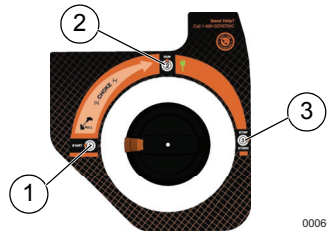
Figure 3-2. Positions du PowerDial
