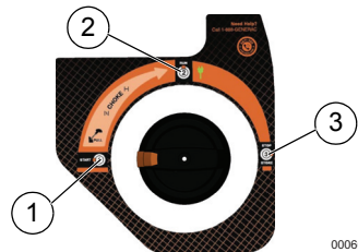
Figura 3-2. Posiciones de PowerDial
