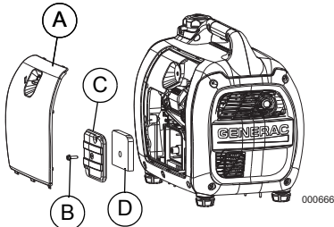
Figure 4-4. Assemblage du filtre à air
